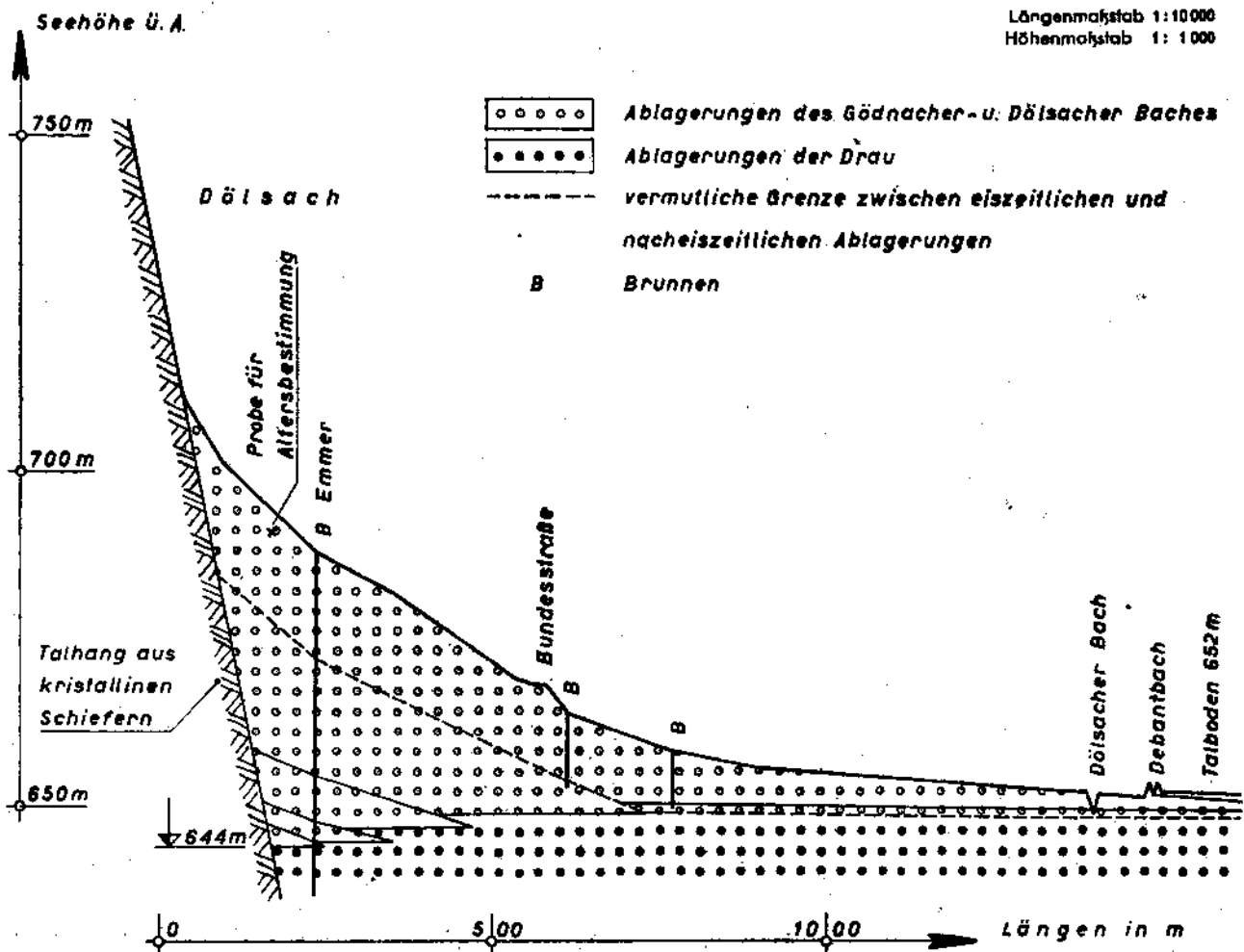
Schematischer Schnitt durch den Schwemmkegel von Dölsach
